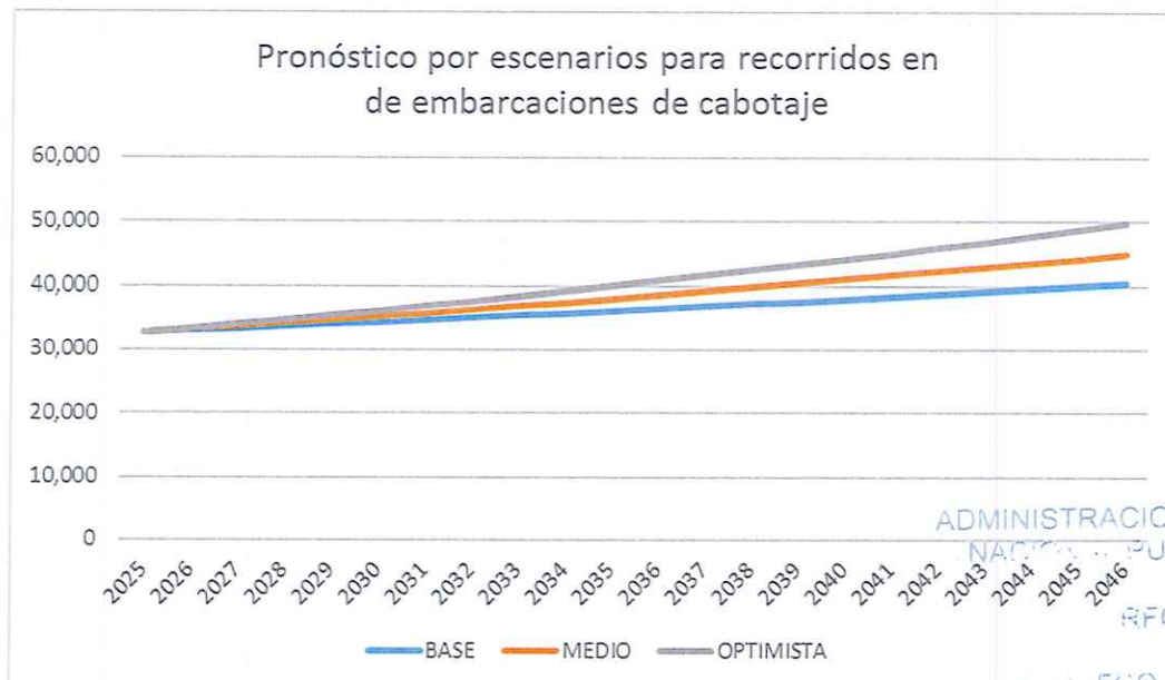
Grafica 20. Proyección de recorridos de cabotaje 2025-2046 por escenarios.
